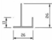
Эф-профиль (3,0м)
